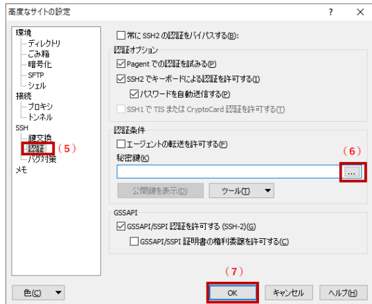
図3 WinSCP 鍵認証設定画面
