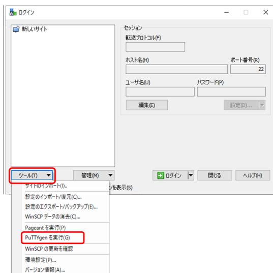
図5 WinSCP 初期設定画面
