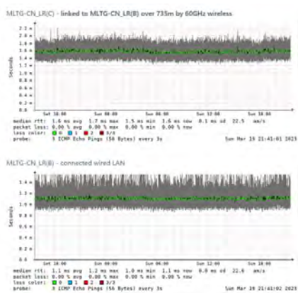
図 5 SmokePing による応答時間計測。
