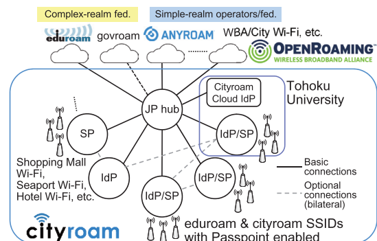
図 2 Cityroam の認証連携ネットワーク概略図。
