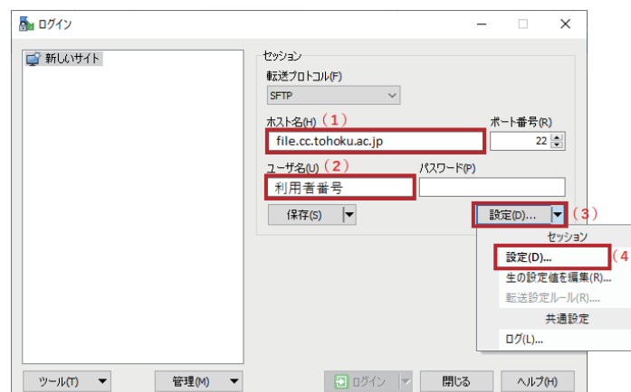
図 2 WinSCP 設定画面
