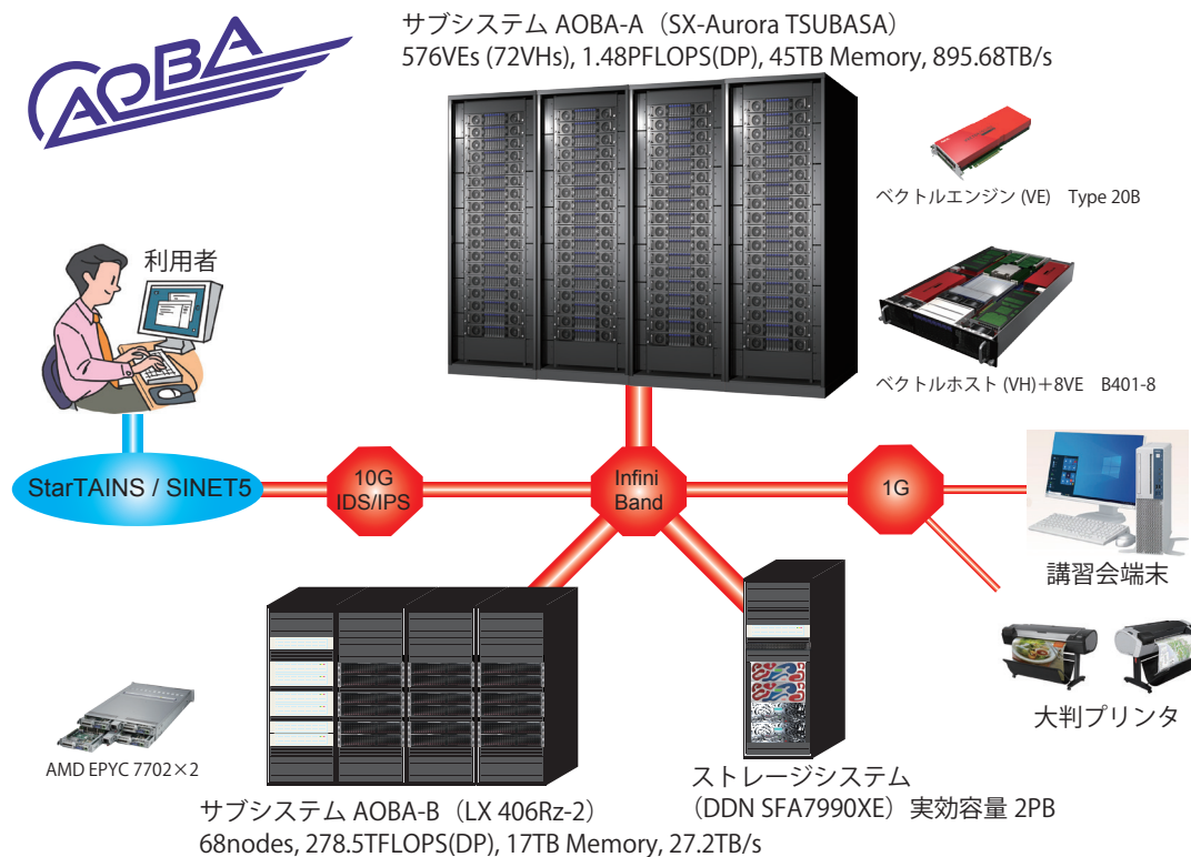
図 1 スーパーコンピュータ AOBA の構成
