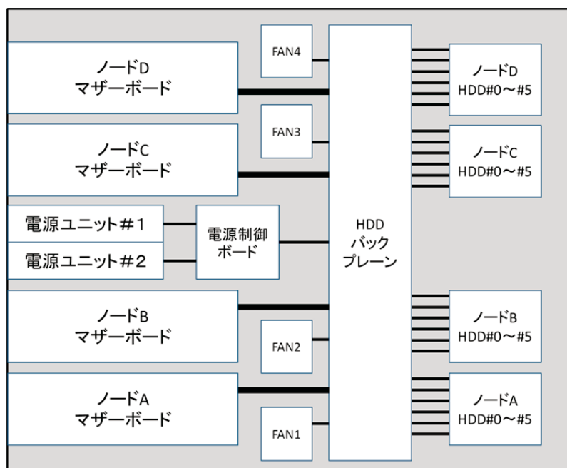
図 1. LX 406Re-2 筐体ハードウェア構成
