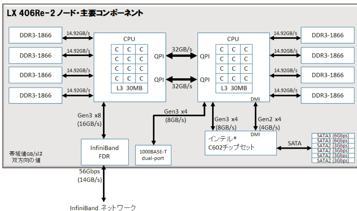
図 4. LX 406Re-2 ノード主要インターフェイス性能
