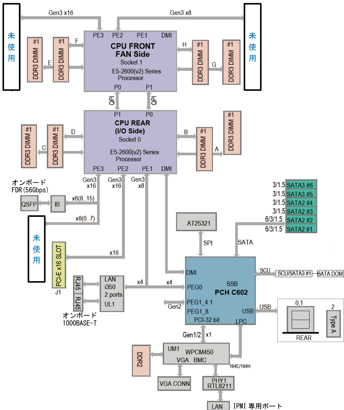
図 2. LX 406Re-2 システムブロックダイアグラム
