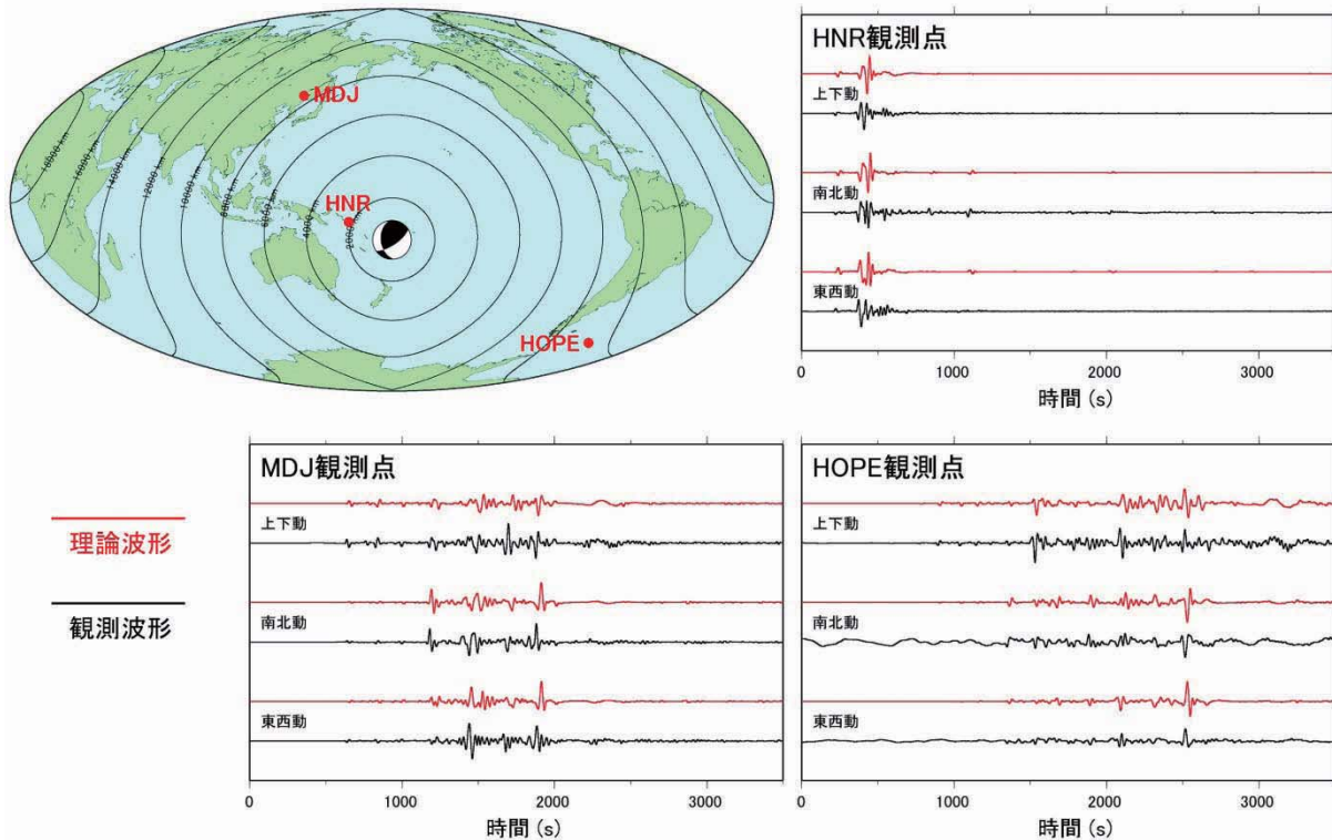
図 3：球座標系 2.5 次元差分法による地球の理論地震波形（赤線）と観測波形（黒線）の比較 [14]。3 観測点それぞれで上下動・南北動・東西動の 3 成分を比較。震源の位置・メカニズムと観測点位置は左上の地図に示した。すべての波形に 1/30 Hz のローパスフィルタを適用。
