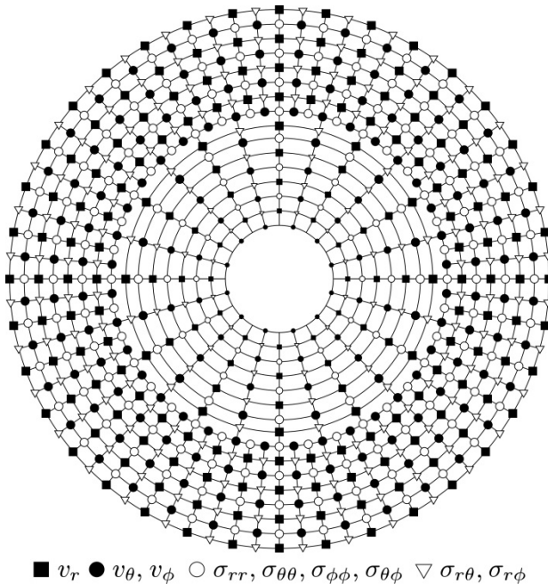
図 2: 計算で用いた差分格子の模式図. 黒が粒子速度, 白が応力の格子を表す.
